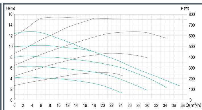
WITA go.max F 65-12F-340
